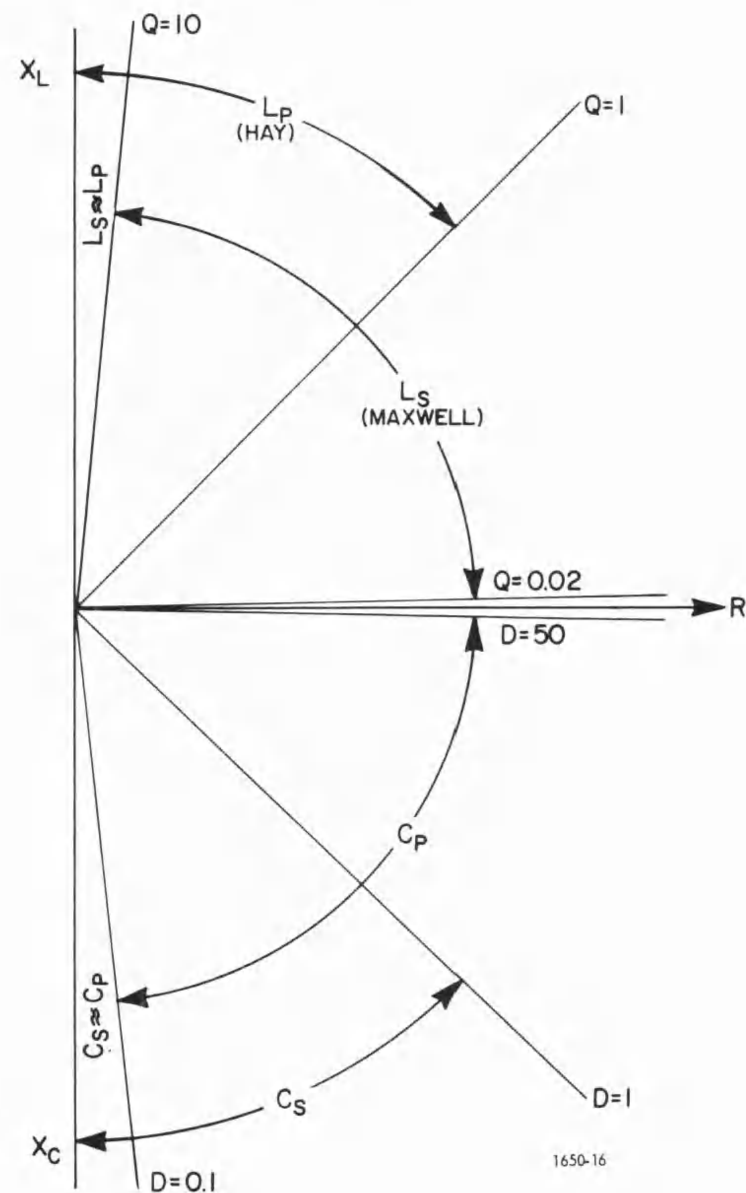
Figure 2-4. DQ coverage chart.
