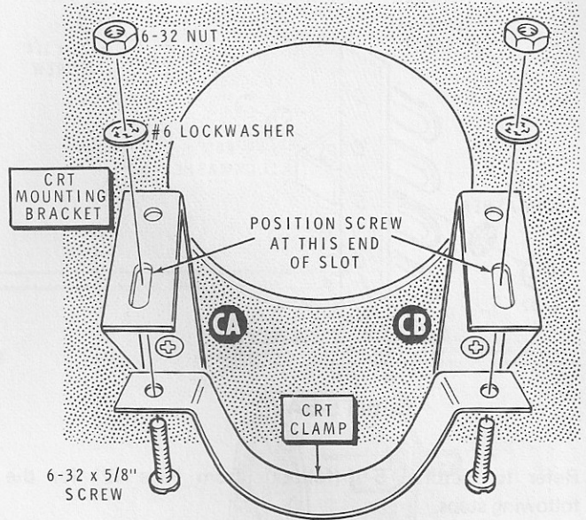
Detail 5-4E
