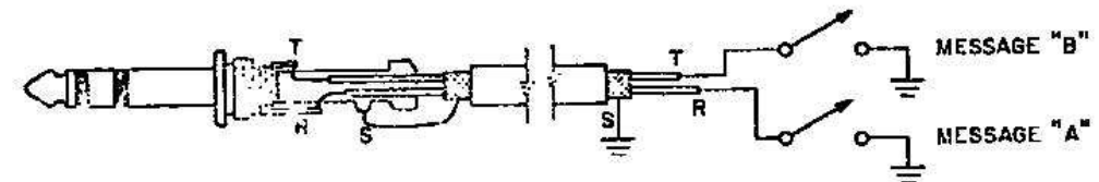
e) I.D. KEY (2-CIRCUIT)
