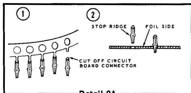
Detail 9A
