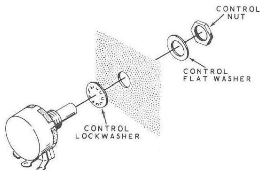
Detail 3E
