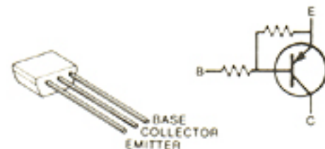
RN2204 Q12, Q18
