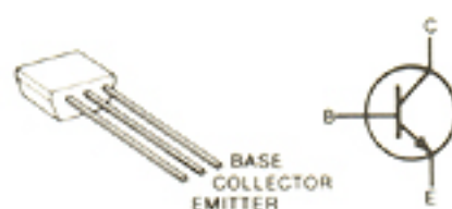
2SC2458 GR Q5, Q6 Q7, Q13
