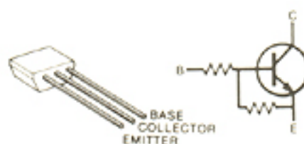
RN1204 Q9, Q11 Q14, Q16 Q17
