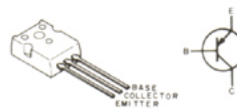
2SA1359 Y Q1
