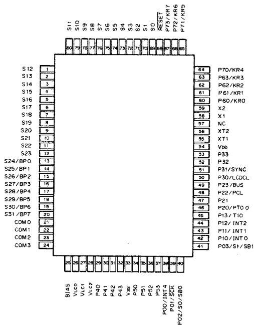
μPD75308GF-101-3B9 IC1 (CPU)
