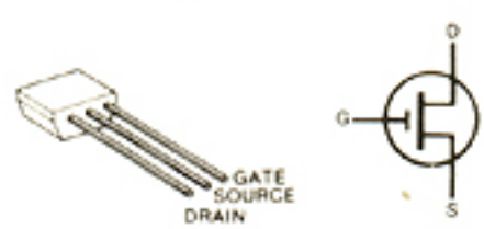
2SK241 Y Q2
