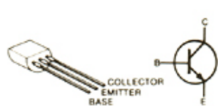
2SC2407 Q15 (UX-29A/E only)
