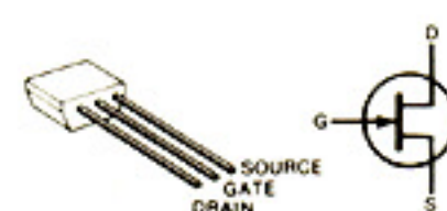
2SK184 Y Q18, Q19
