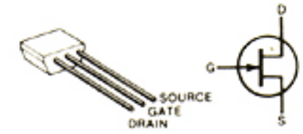
2SK184 Y Q18, Q20, Q21
