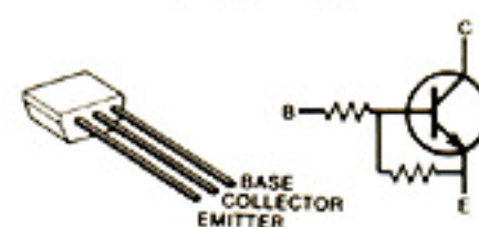
RN1204 Q14, Q33, Q34
