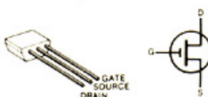
2SK241 Y Q3
