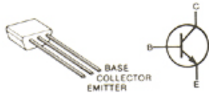
2SC2458-GR
