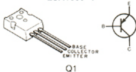
2SA1359 Y
