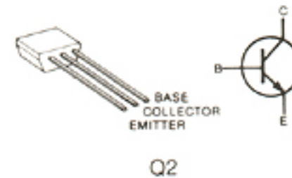
2SC2458-GR
