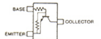
UN9211 (Symbol: 8A)
