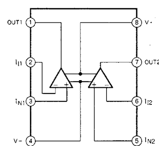
IC3 \mu PC358G2
