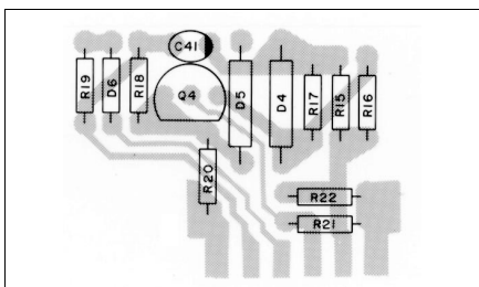
406-973-A TOP
