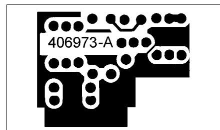
406-973-A BOTTOM
