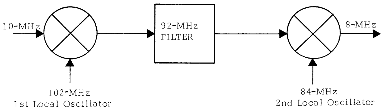
3020A Mixer Scheme.
