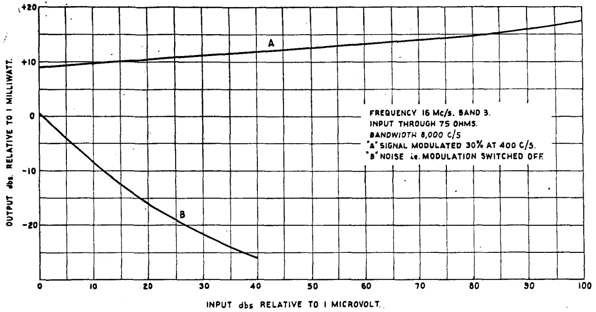
FIG. 15. AGC RESPONSE.
