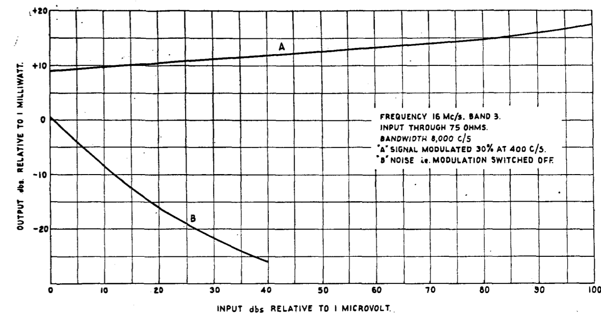
FIG. 15. AGC RESPONSE.
