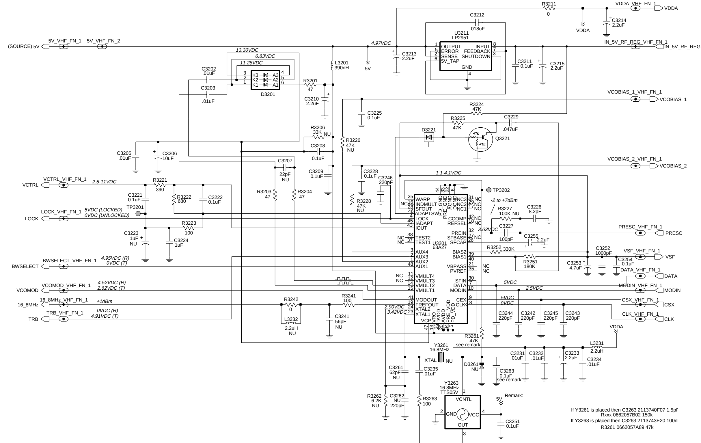
VHF (136-174 MHz) FRACN
