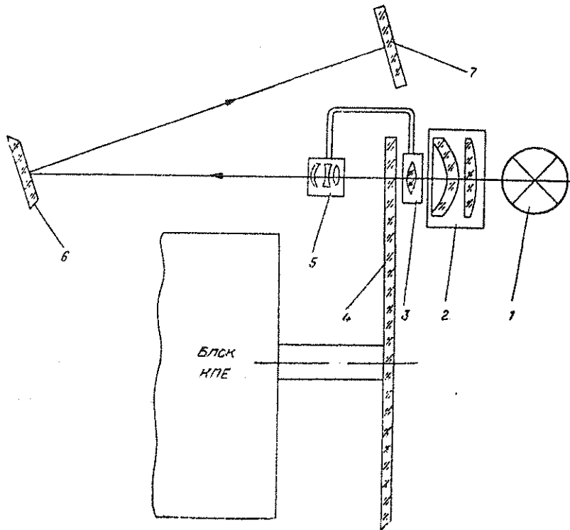
Рис. 4. Схема проектирования изображения микрофотошкалы на экран: 1 — лампа освещения; 2 — конденсор; 3 — подвижная линза; 4 — микрофотошкала; 5 — объектив; 6 — зеркало; 7 — экран.
