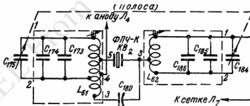
Рис. 8. Кварцевый фильтр.
