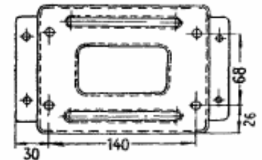
РАМА ВЫПРЯМИТЕЛЯ
