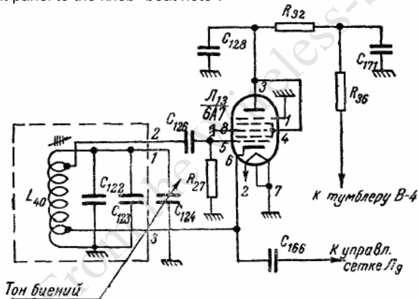
Рис. 11. Второй гетеродин
