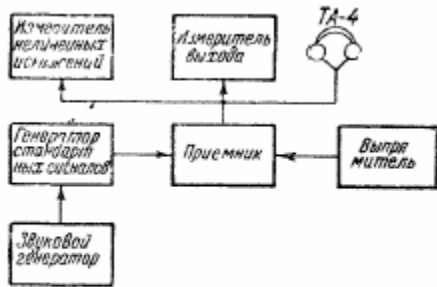
Рис. 28. Блок-схема измерения коэффициента нелинейных искажений.
