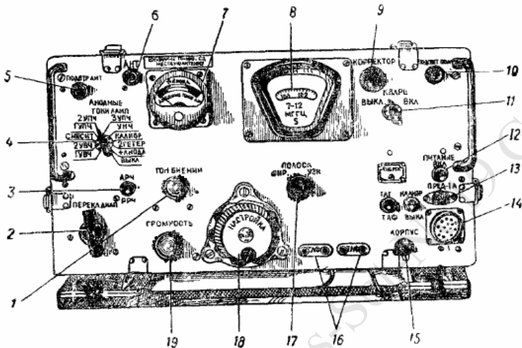
Рис. 16. Передняя панель:
