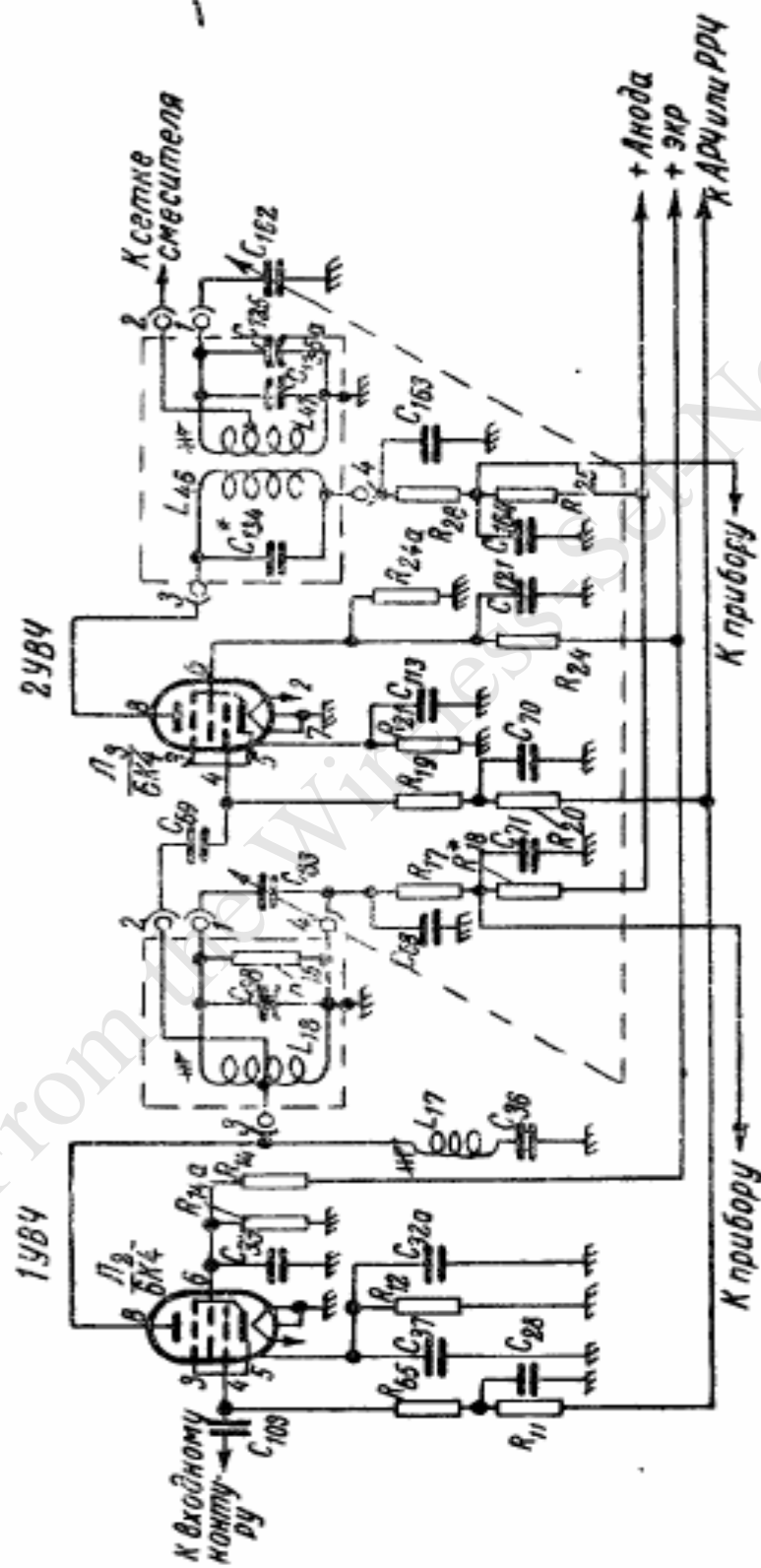
Рис. 30. Усилитель высокой частоты до изменения.
