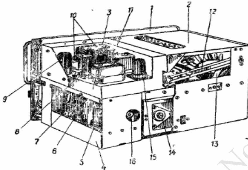
Рис. 15 Вид радиоприемника без кожуха. 1—передняя панель; 2—блок В. Ч; 3—блок П. Ч; 4—блок Н. Ч; 5—лампа L_{11} ; 6—лампа L_{12} ; 7—лампа L_{13} ; 8—лампа L_6 ; 9—лампа L_7 ; 10—фильтр промежуточной частоты, 11—лампа L_8 ; 12—тяга под- стройки антенны; 13—барабанный переключатель; 14—блок конден- саторов переменной емкости; 15—лампа L_{16} ; 16—контур 2-го гете- родина
