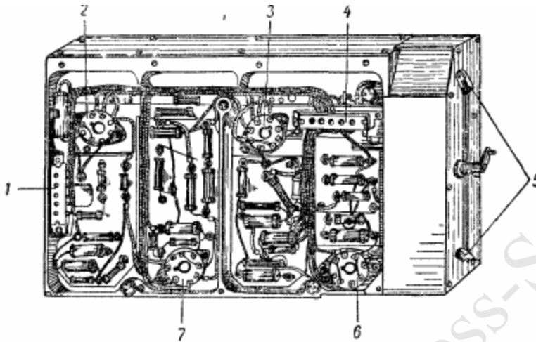
Рис. 21 Блок «ПЧ»: 1—штепсельный разъем; 2—лампа Л 10 ; 3—лампа Л 8 ; 4—штепсельный разъем; 5—конденсаторы С 178 и С 184 ; 6—лампа Л 7 ; 7—лампа Л 9 .
