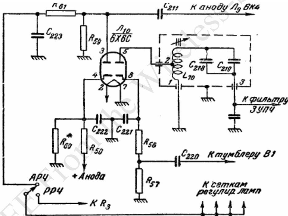
Рис. 9. Детектор сигнала и детектор АРС.
