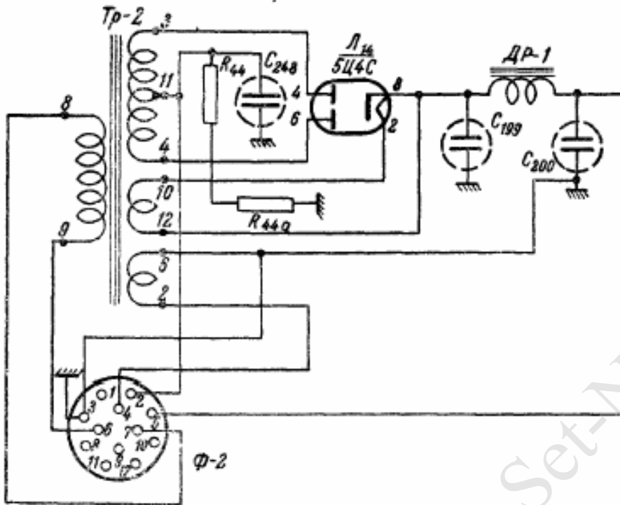
Рис 11 Схема выпрямителя
