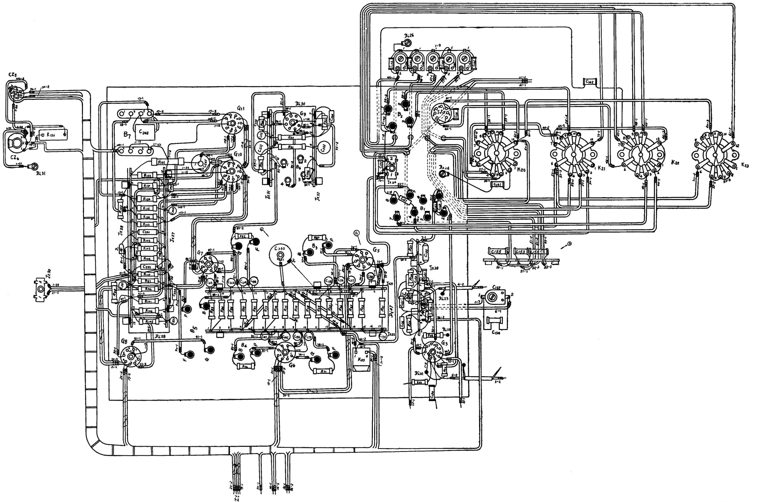
8. 联合单元接线图
