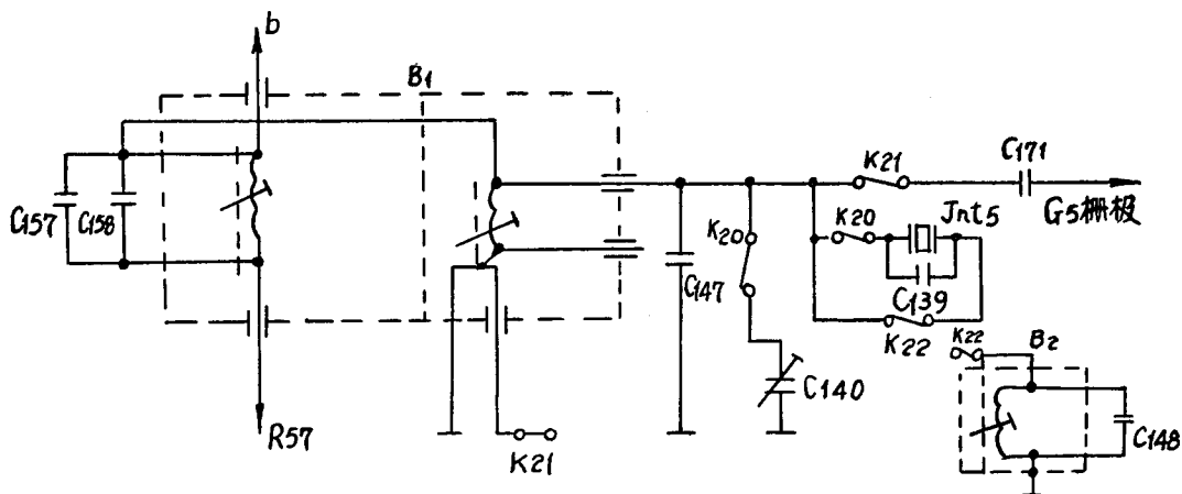
图 4 晶体滤波器电原理图，通带 6 千赫
