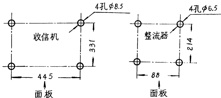
图 8 安装尺寸
