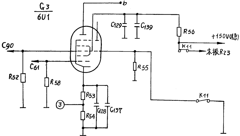
图 2 混频电路，开关 K_{11} 在“调谐”位置
