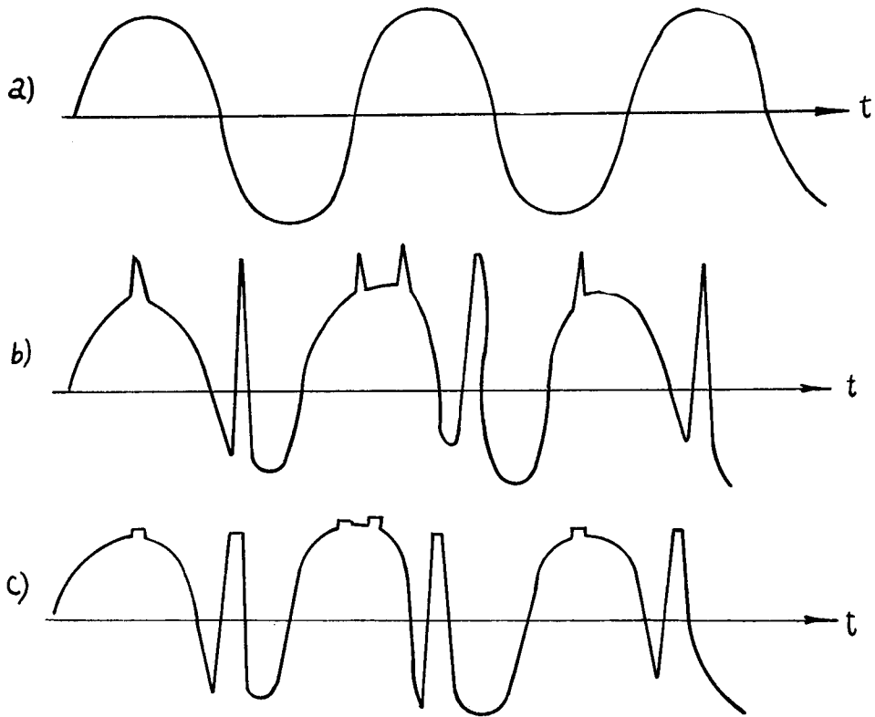
图 9 噪声抑制器电压波形的图解
