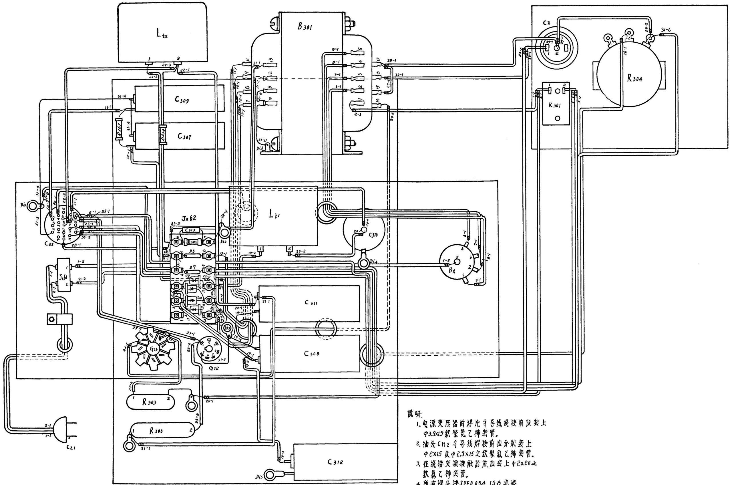
10. 整流器接线图
