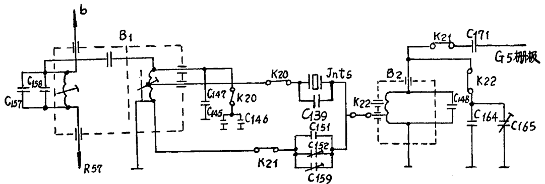
图 7 晶体滤波器电原理图，通带 0.4 千赫
