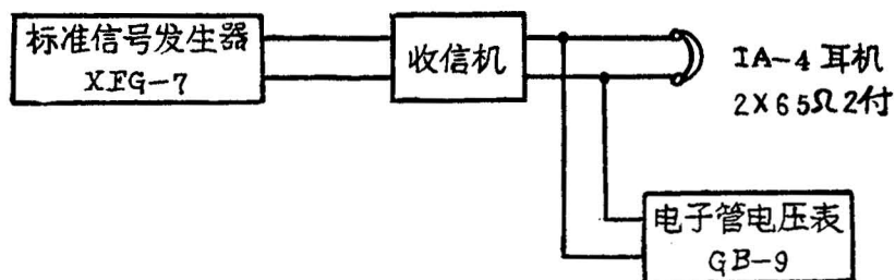
图 16 划分波段与统调高频放大器方框图
