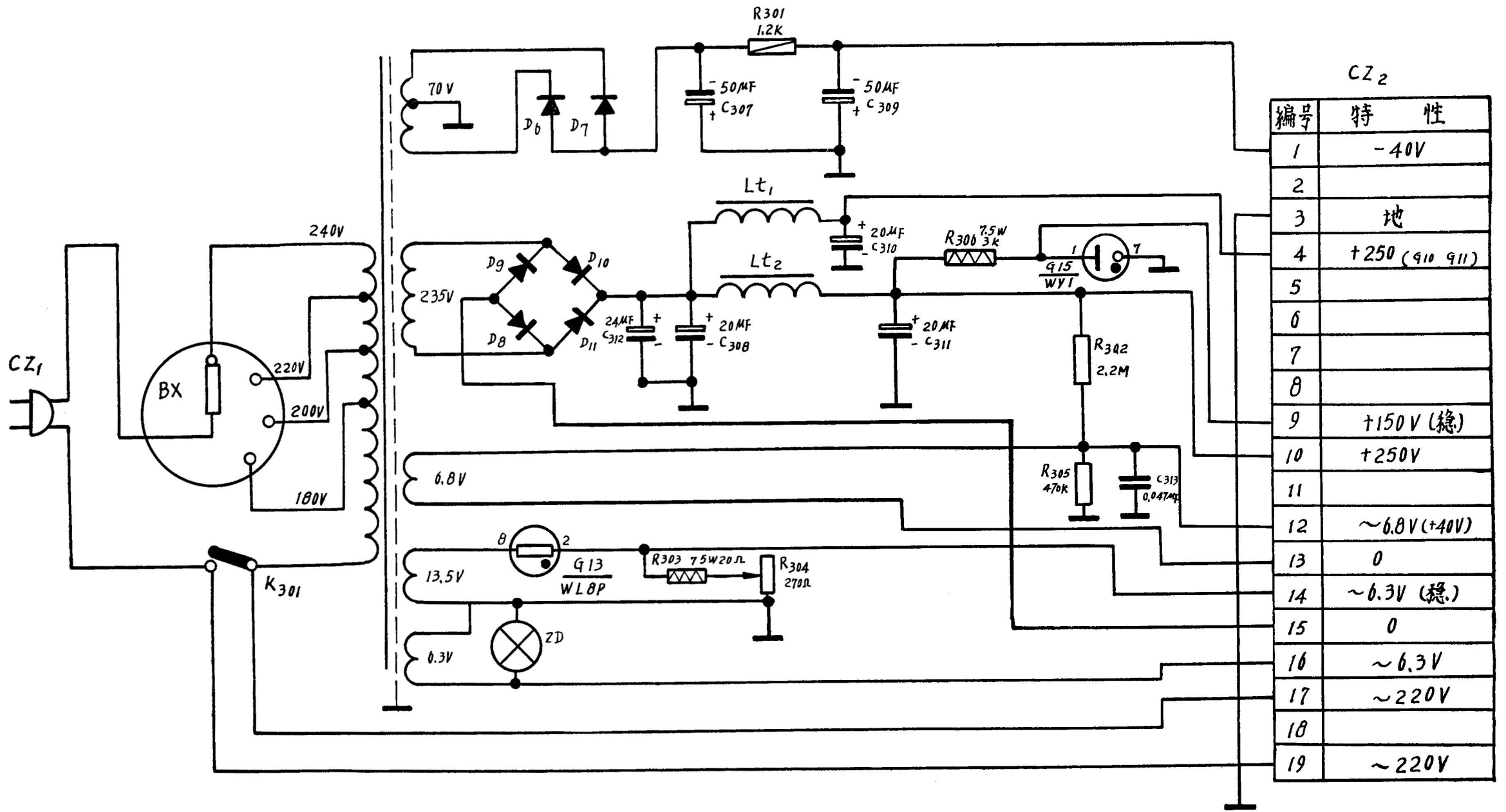
4. 整流器电原理图
