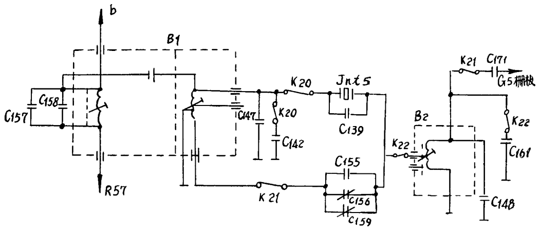
图 5-1 晶体滤波器电原理图，通带 3 千赫
