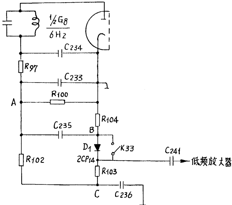
图 8 噪声抑制电路
