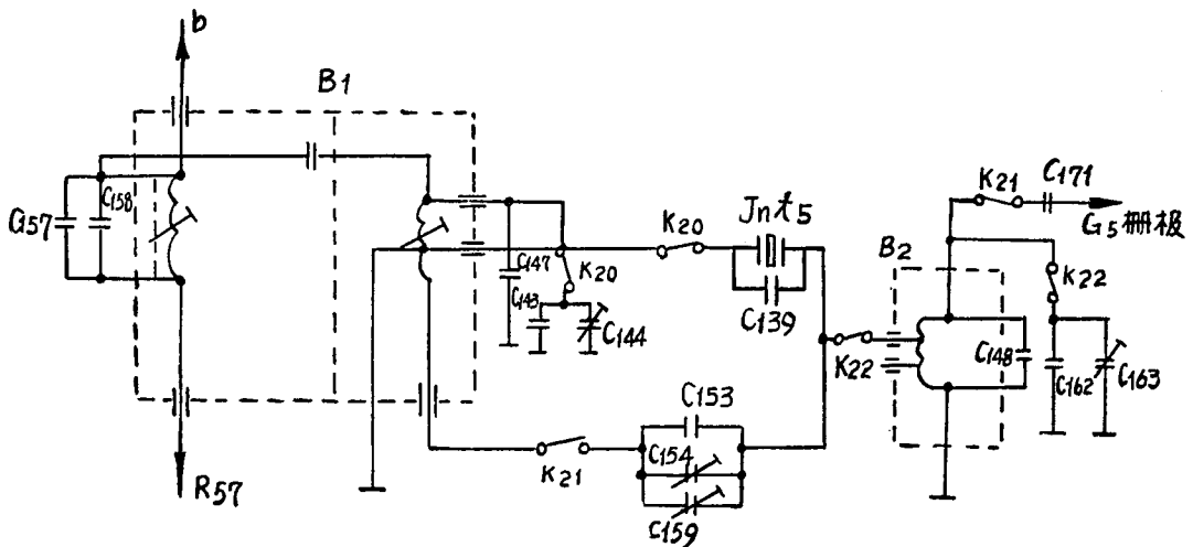
图 6 晶体滤波器电原理图，通带 1.5 千赫
