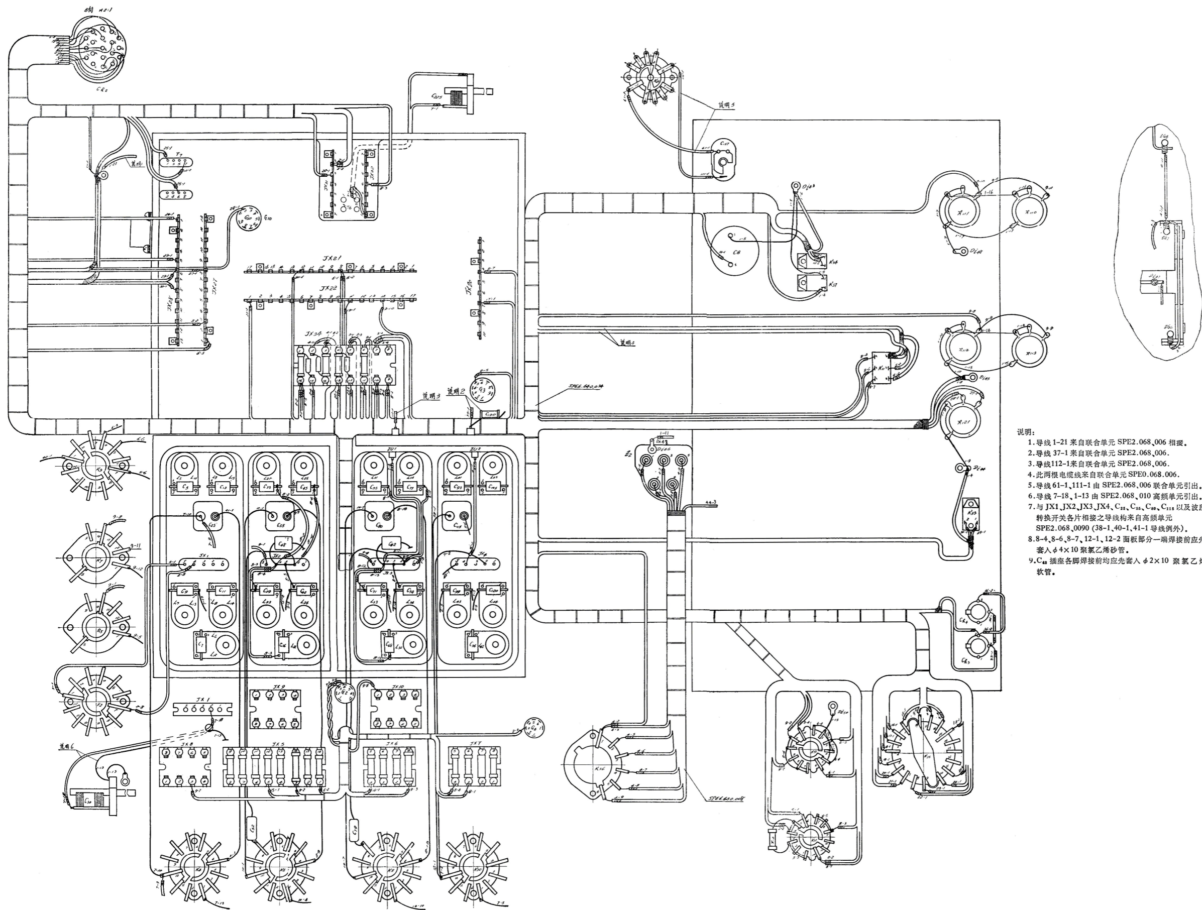
9. 收音机接线图
