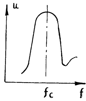
图 5-6 C_H > C_0
