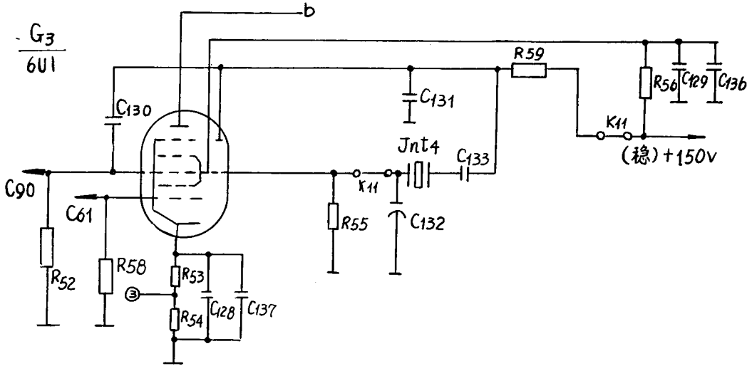
图 1 晶体振荡变频电路，开关 K_{11} 在“晶体”位置
