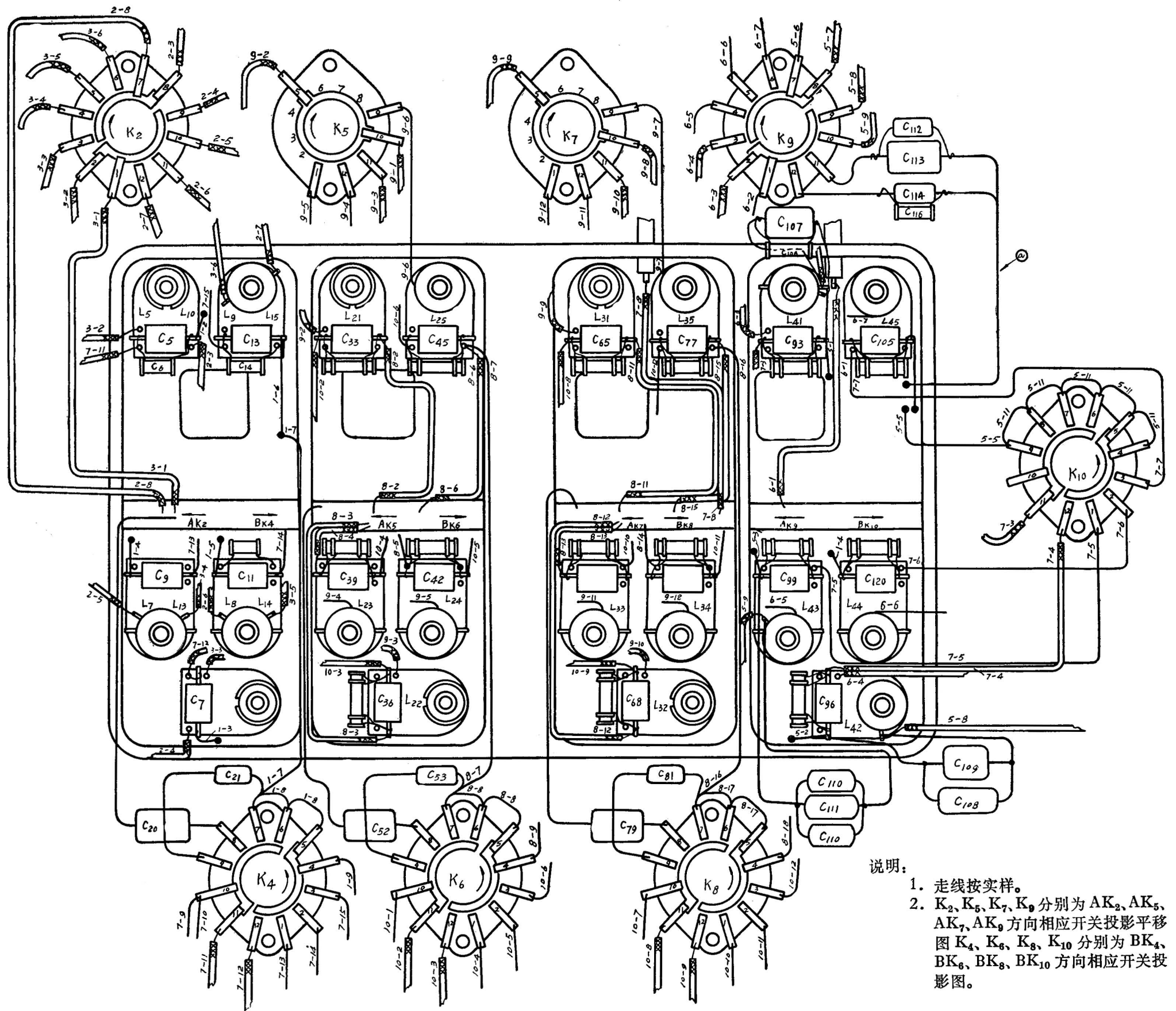
7. 高频单元 B 接线图
