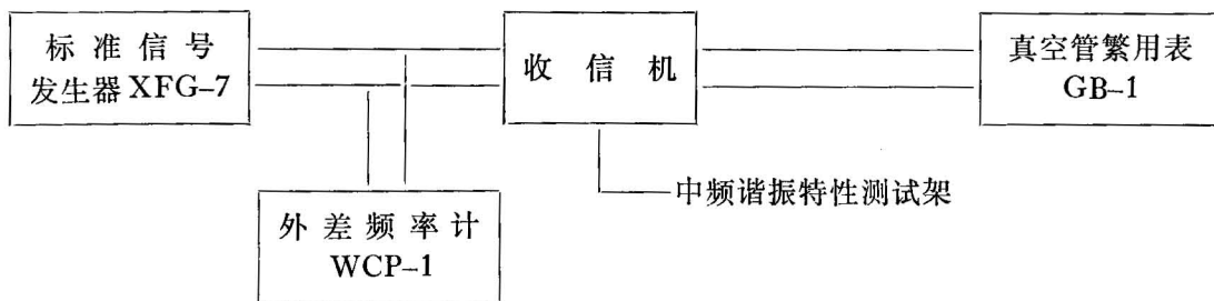
图 15 调整中频谐振特性方框图
