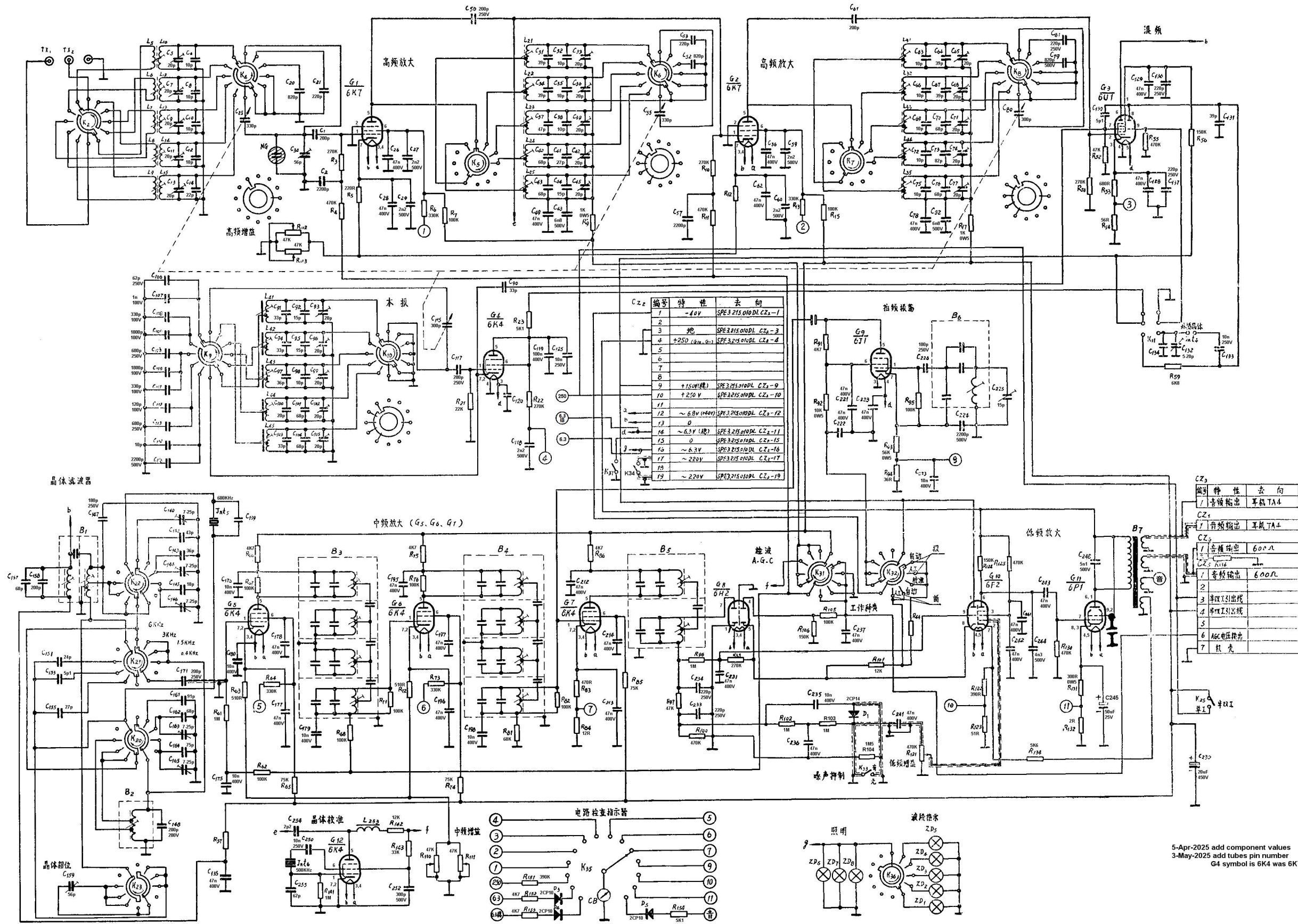
5. 收音机电原理图
