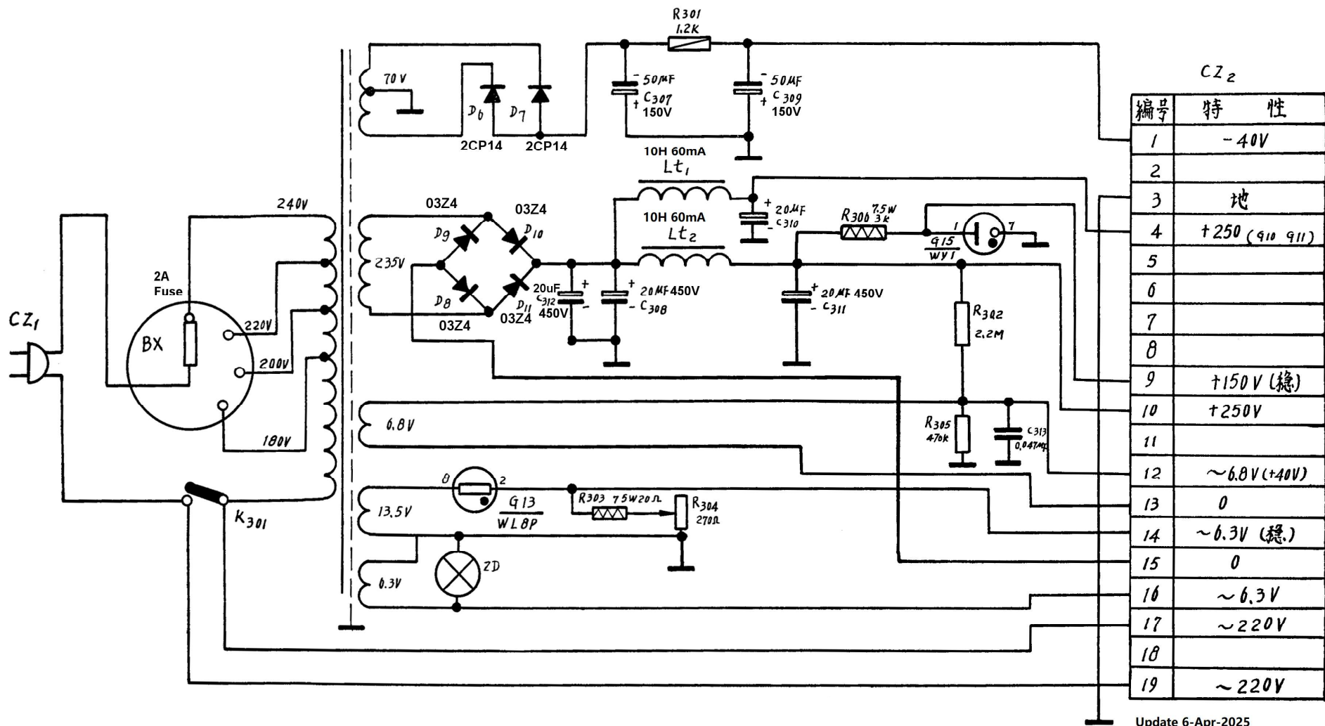
4. 整流器电原理图
