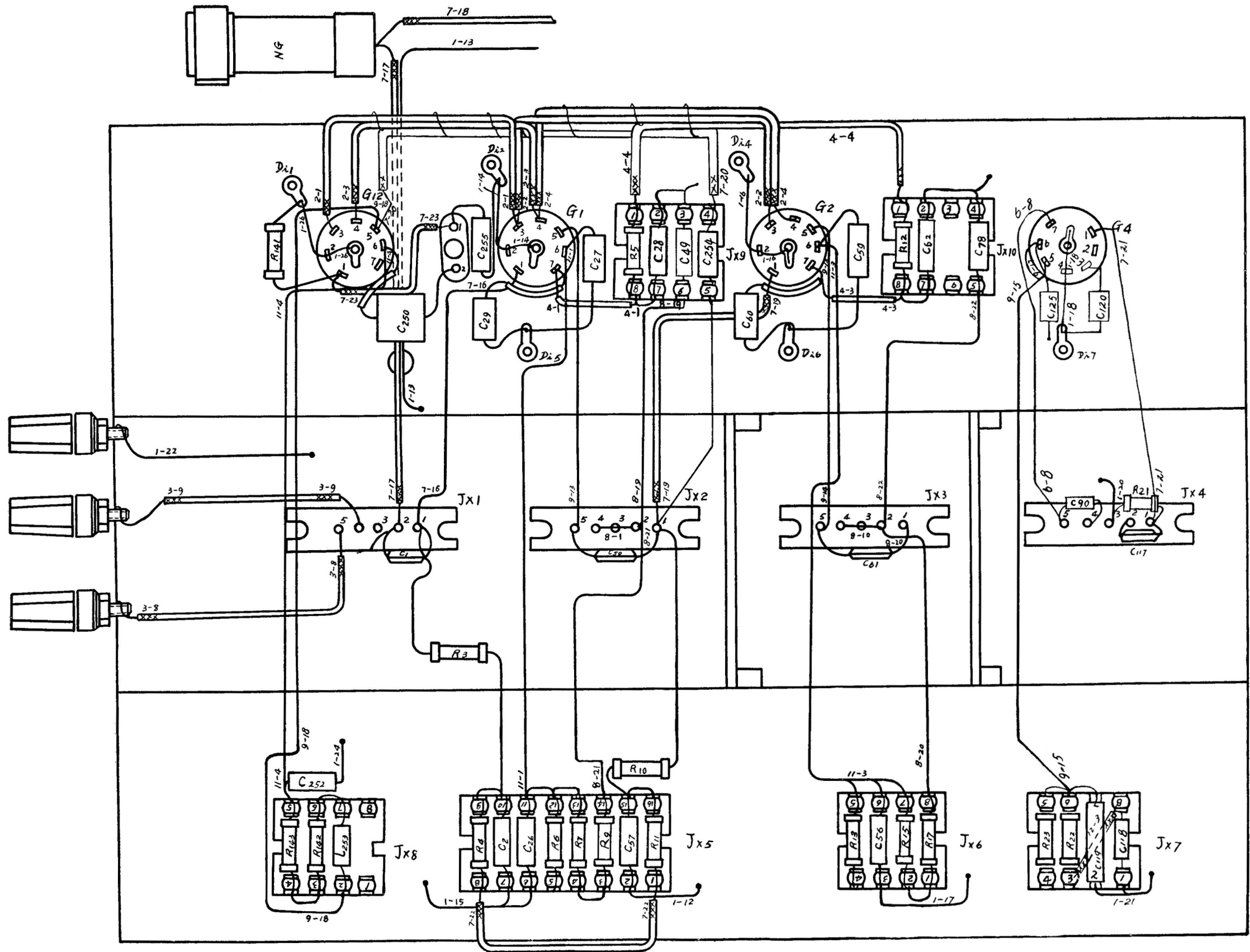
6. 高频单元 A 接线图
