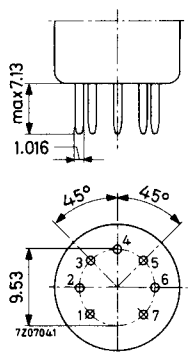
MINIATURE 7-PIN BASE (IEC 67-1-10a)
