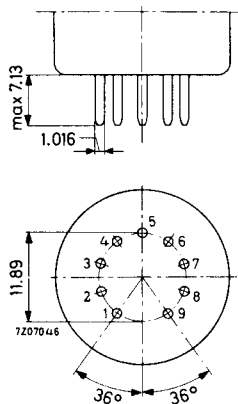
NOVAL BASE (IEC 67-I-12a)
