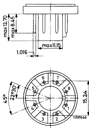
NEO EIGHTAR BASE (IEC 67-1-31a)
