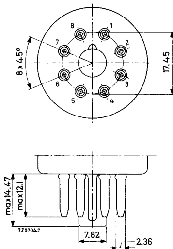
OCTAL BASE (IEC 67-1-5a)
