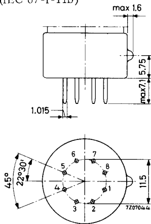
RIMLOCK BASE (IEC 67-1-11b)
