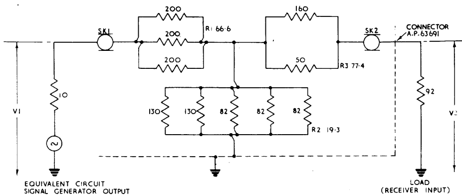
ATTENUATOR A.P. 63693 FIG. 1
