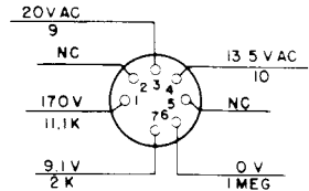
3D MIXER V205 6C4
