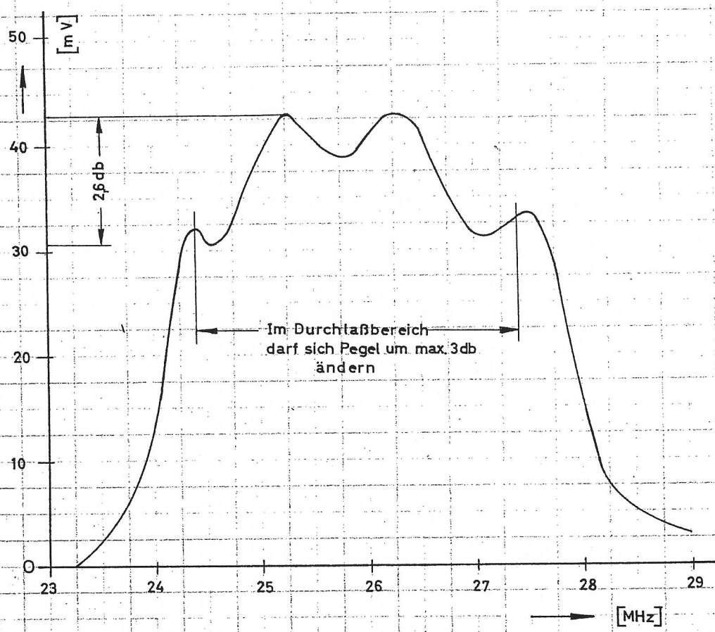
24,4 - 27,4 MHz - Filter (nur im V. Bereich)
