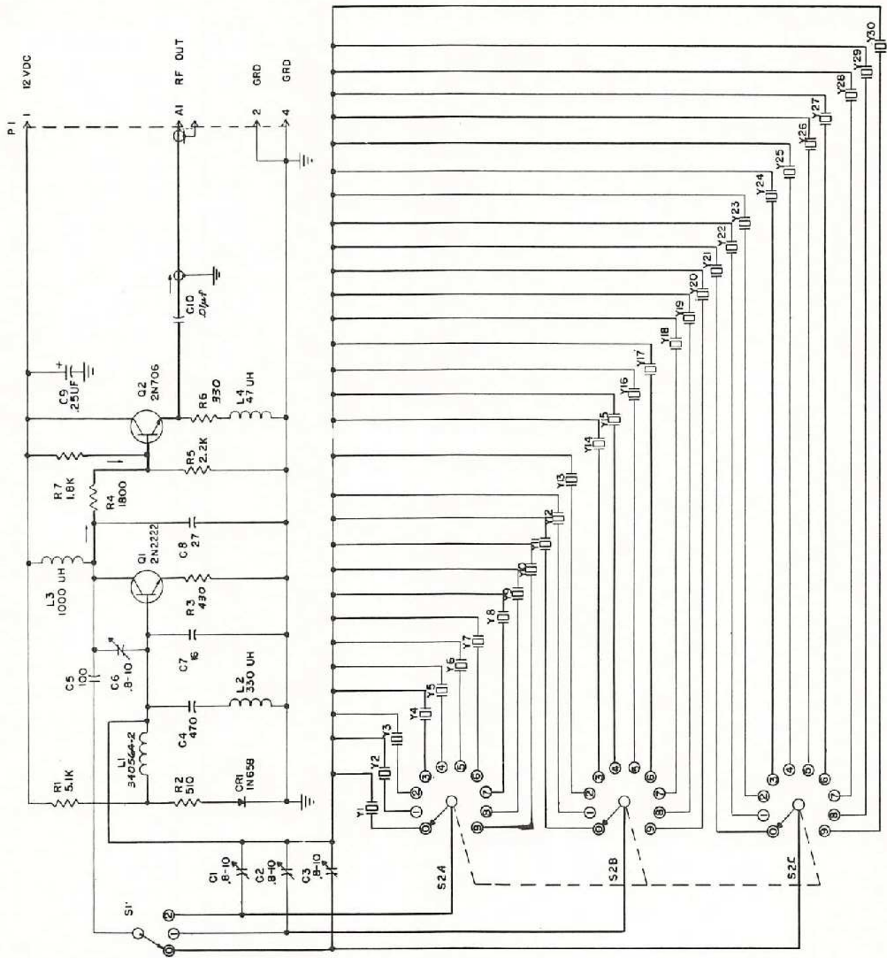
Figure 7-1. CS-224 Schematic Diagram
