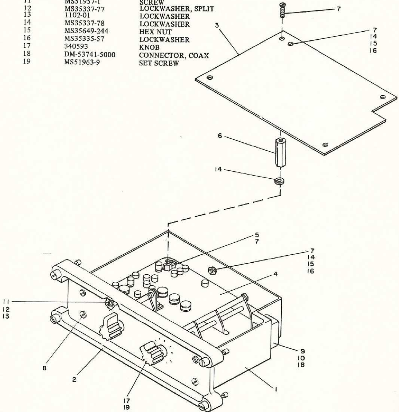
Figure 7-2. CS-224 Crystal Selector
