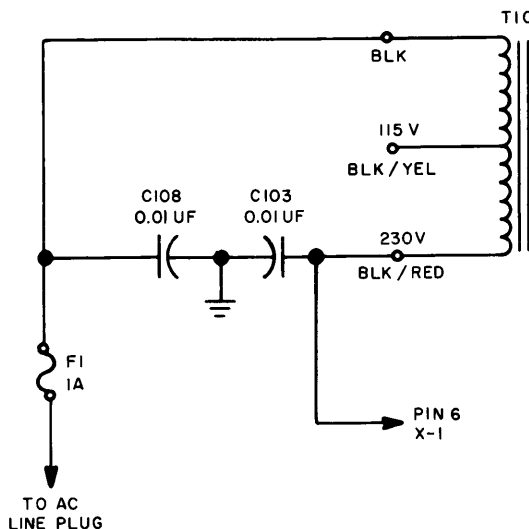
230 VOLT OPERATION
