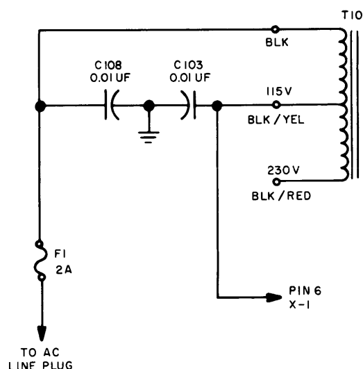
115 VOLT OPERATION
