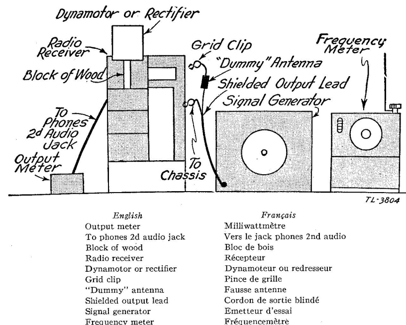
FIGURE 19.—Radio-récepteur BC-312-( ); disposition de l'équipement d'essai pour l'alignement en utilisant un milliwattmètre.
