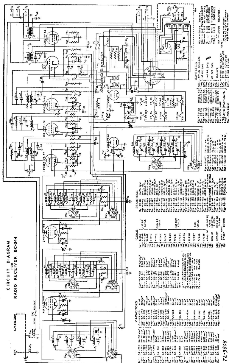
FIGURE 28.—Radio-récepteur BC-344, schéma comprenant la liste des pièces.
