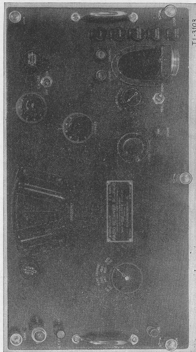
FIGURE 3.—Radio récepteur BC-314-C, vue du panneau antérieur.
