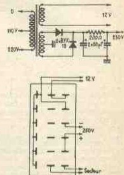
Fig. 2. — Schéma de principe de l'alimentation du BC 603 et câblage du bouchon d'alimentation (intérieur du boîtier commutateur).
