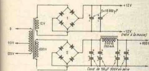
Fig. 4. — Schéma de principe de l'alimentation du BC 604 : 1 = redresseur sec au sélénium 12 V - 3 A (matériau) ; 2 = pont réalisé avec 4 diodes BYX 10
