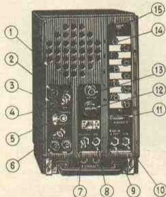
Fig. 1. — Les différentes commandes sur la face avant du BC 603 : 1. Capot de protection pouvant s'enlever ; 2. Fusible à remplacer par un voyant marche-arrêt ; 3. Fusible à remplacer par un interrupteur AM-FM ; 4. Marche-arrêt du haut-parleur ; 5. Poussoir levé ; 6. Potentiomètre permettant de régler le niveau de coupure du « squeal » ; 7. Interrupteur permettant le réglage exact sur la station ; 8. Arrêt-marche des sorties câbles ; 9. Arrêt-marche du « squeal » ; 10. Arrêt-marche du C.V. pour la recherche des stations ; 11. Potentiomètre de volume ; 12. Voyant qui s'allume en présence d'une émission, en position « squeal » ; 13. Touches à appuyer pour obtenir l'accord exact immédiat sur une station pré-régulée ; 14. Orifice pour l'accord ; 15. Orifice pour l'accord (se régler au préalable en bout de l'accord côté 30 MHz).
