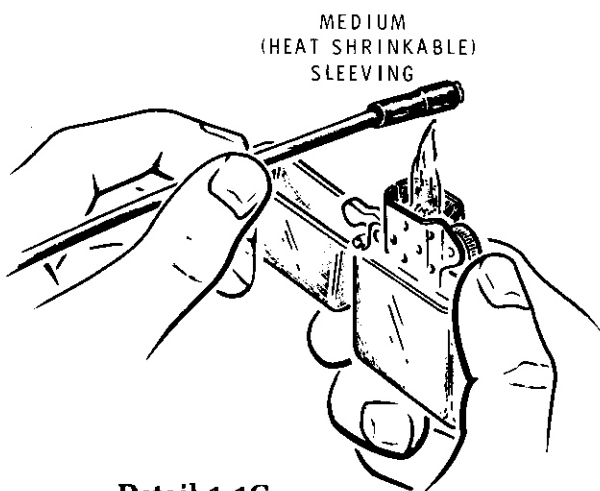
Detail 1-1C
