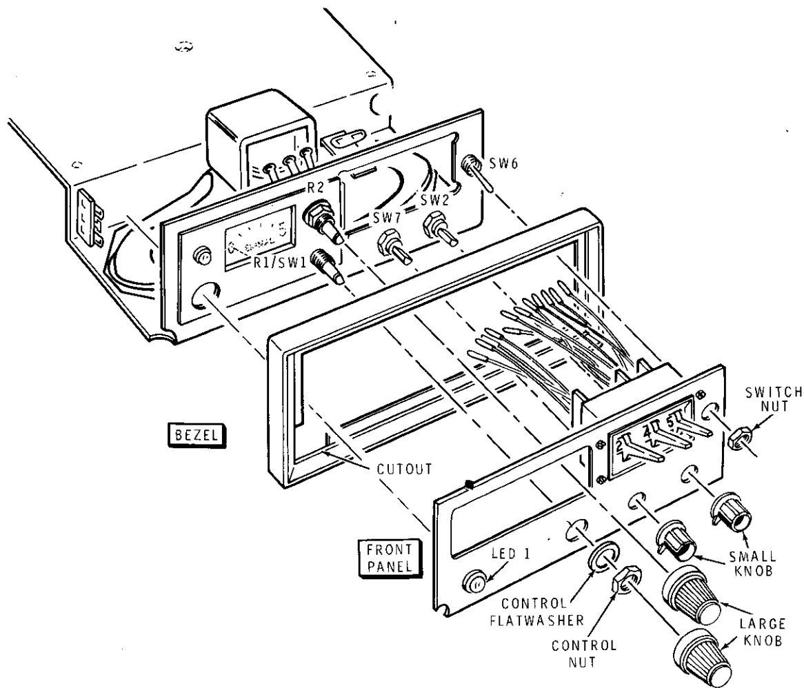
Detail 1-8A
