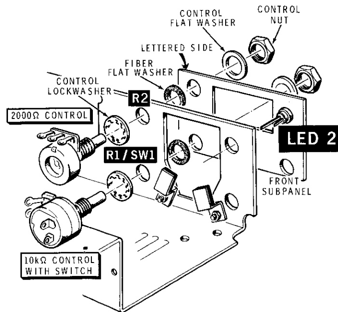
Detail 1-3E
