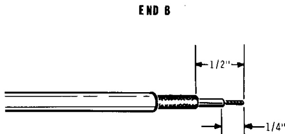
Detail 2-7E
