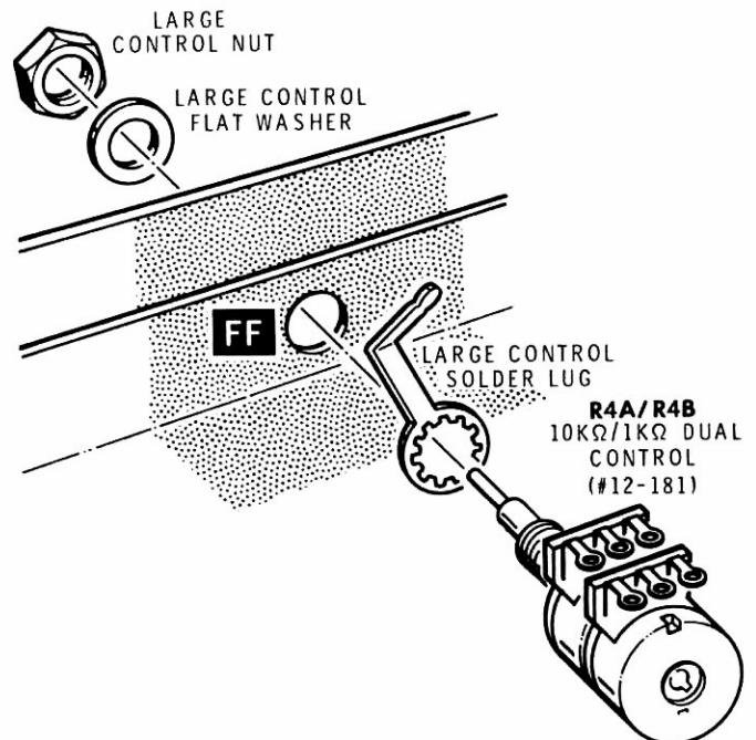
Detail 15-4C
