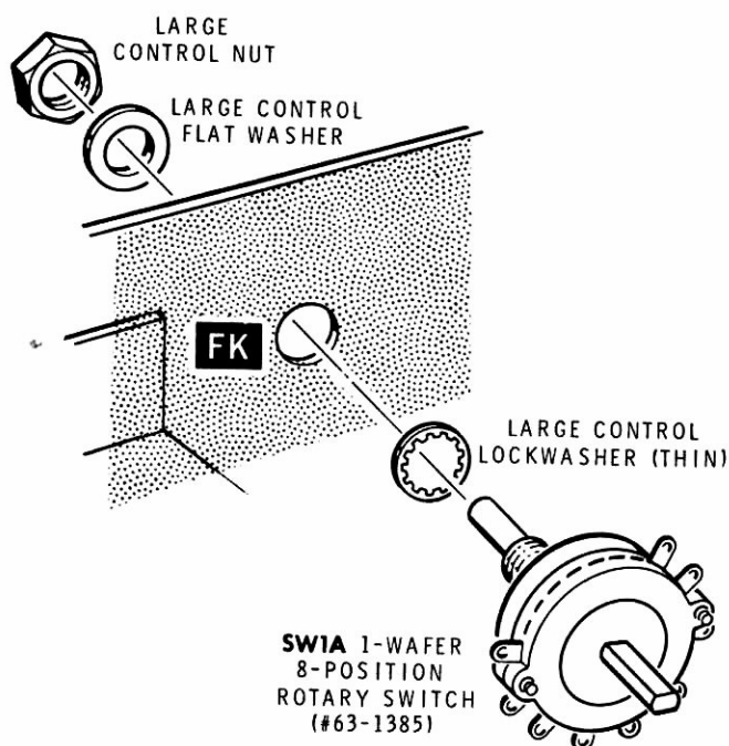
Detail 15-4E
