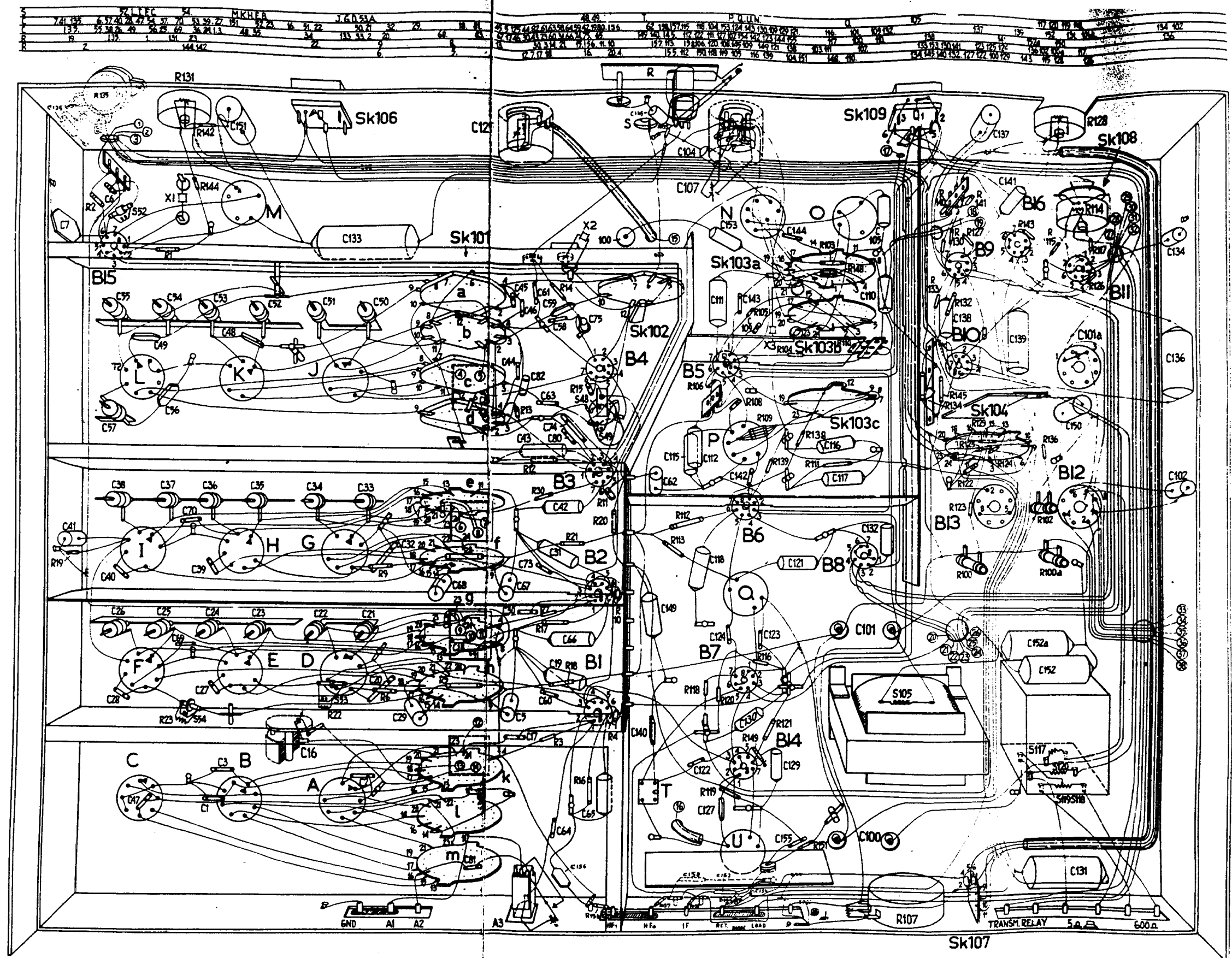
FIG. 14 BEDRADING (ONDERZUDE CHASSIS)
