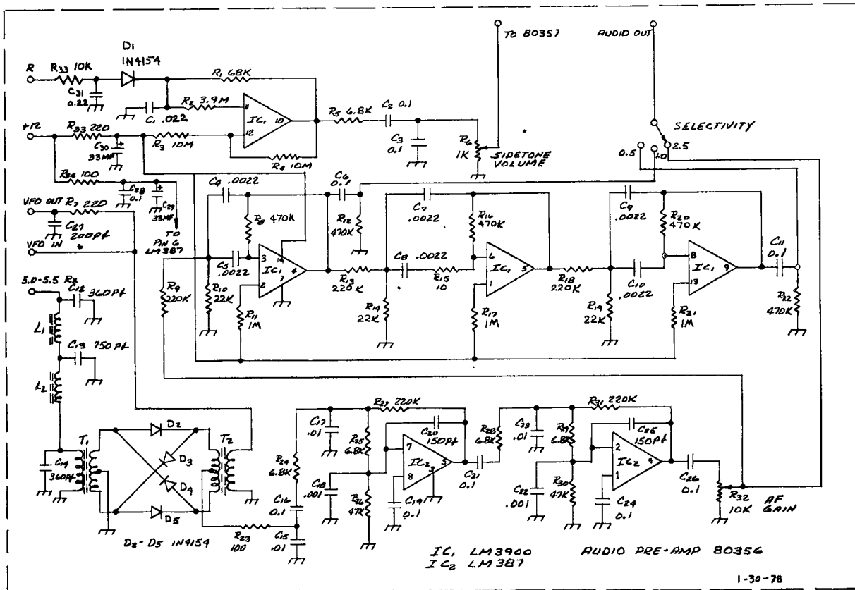
AUDIO PRE-AMP 80356
