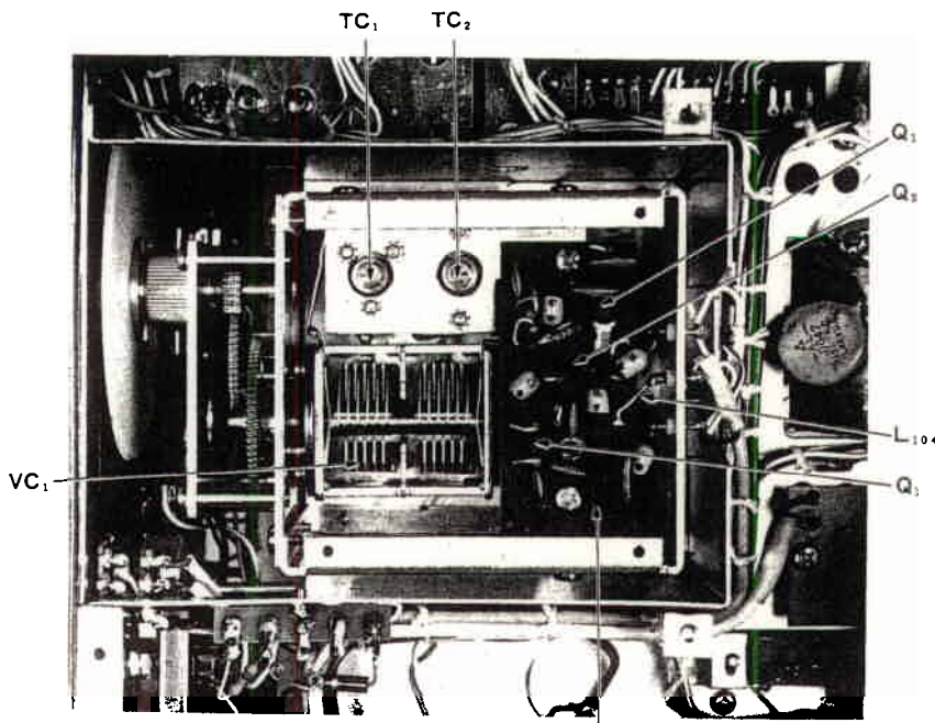
VFO(PB-1307)
