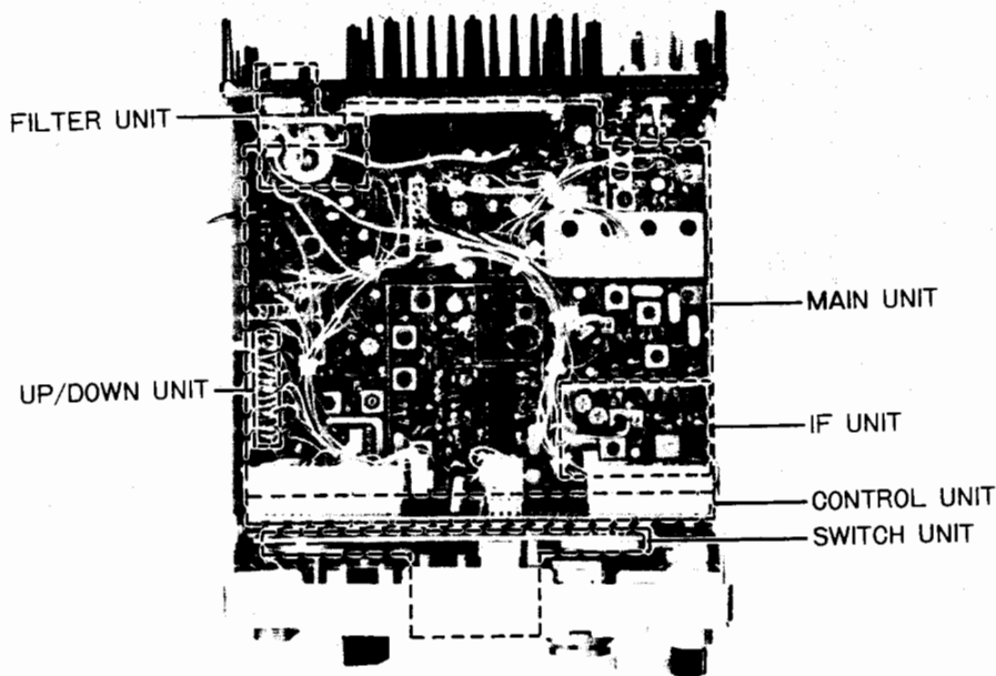
ユニット配置図 (底面側)
