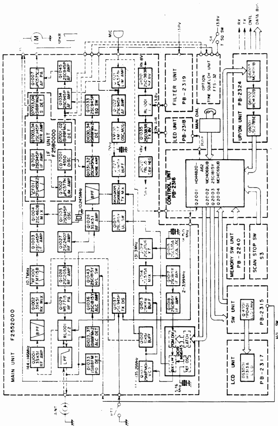
第1図 ブロックダイアグラム
