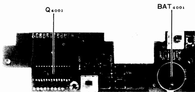
スイッチ基板ユニット
